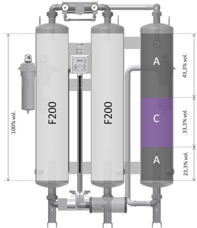
Füllung Trocknerbehälter: F200 Aluminiumgel Füllung dritter Behälter: A = Aktivkohle C = Katalysator
