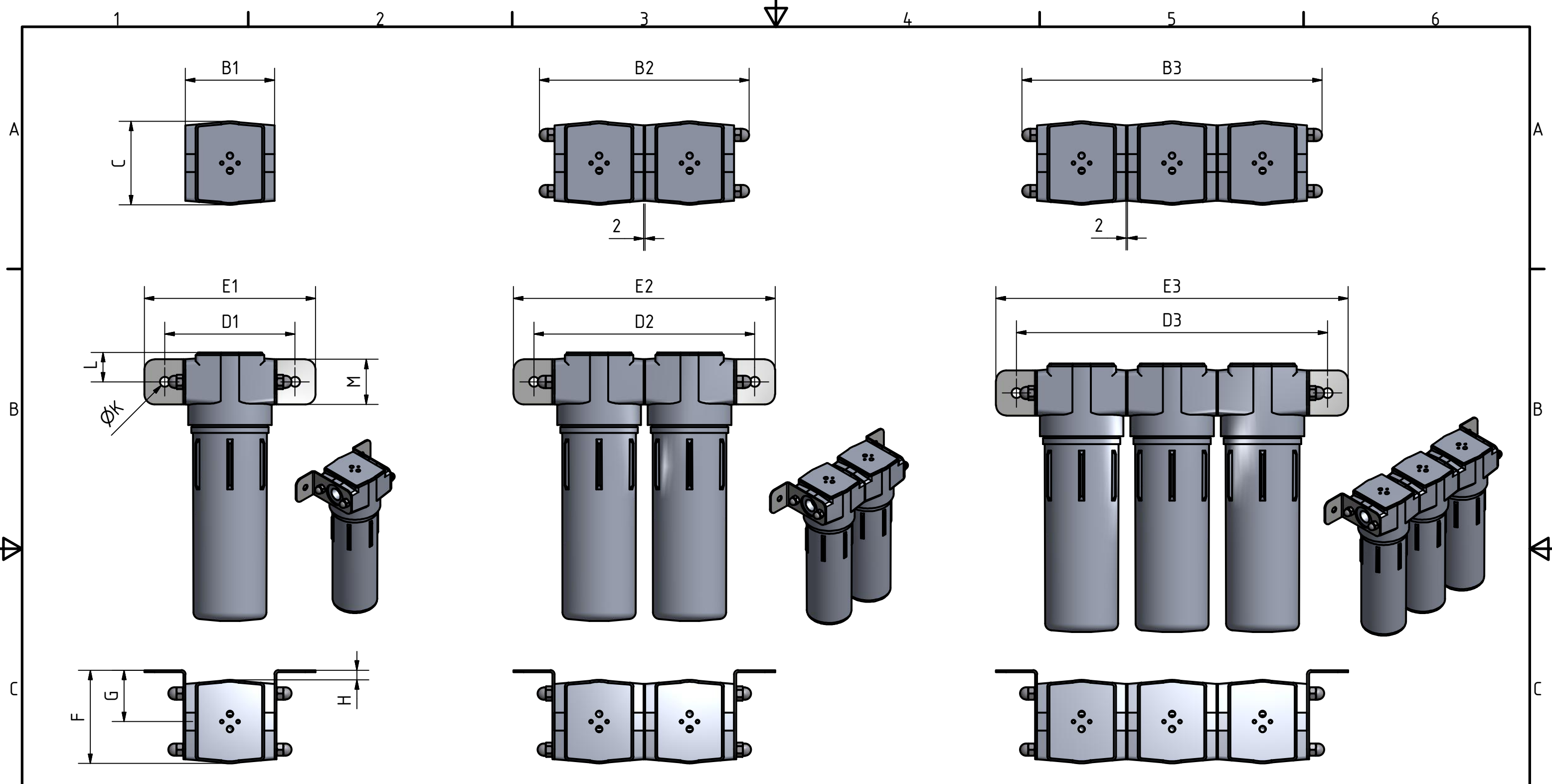
Abmessungen / Dimensions ( in mm )
